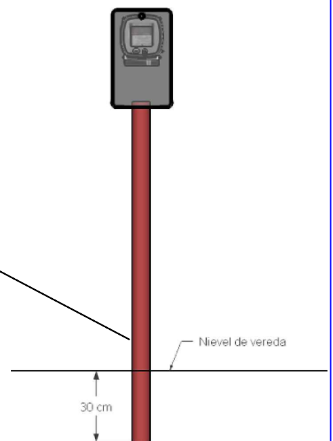
Dimensiones del pilar simple
